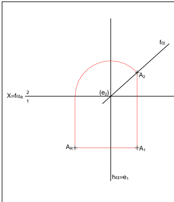
Rebatimento de um plano de topo em torno do seu traço horizontal
